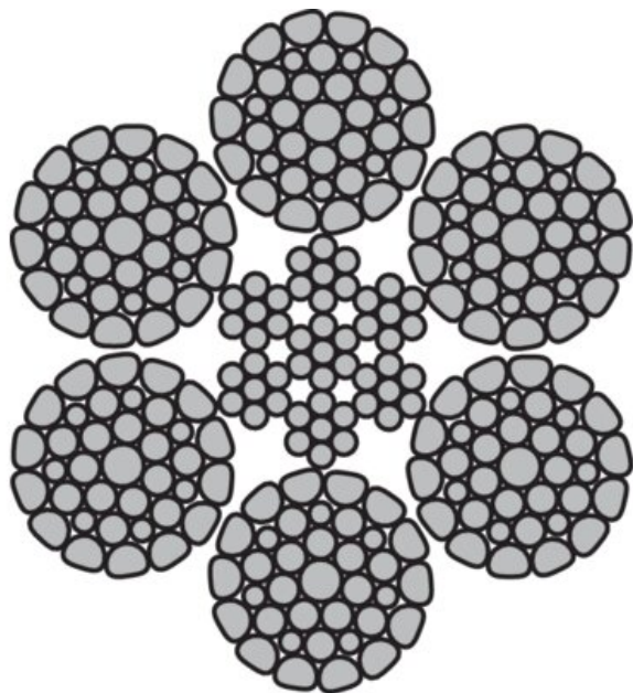
Въже за телфер
